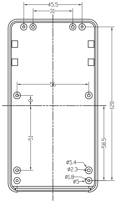
上盖底视图
