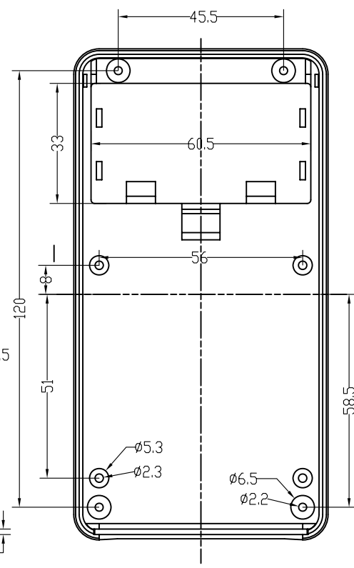
下盖正视图
