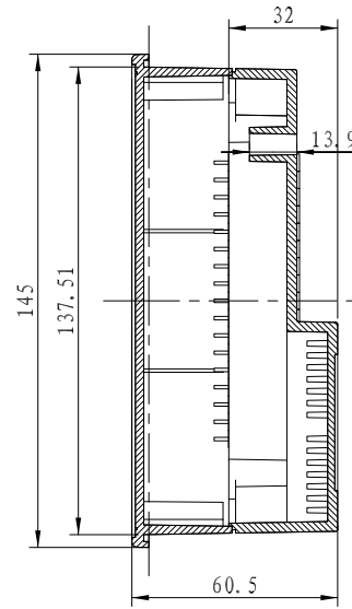
剖面 A-A
