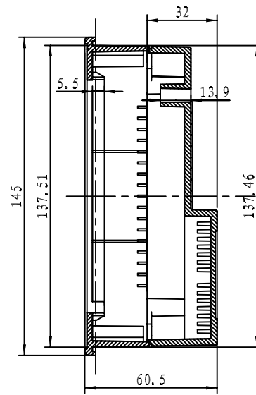
剖面 A-A
