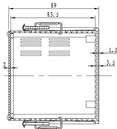
剖面 A-A
