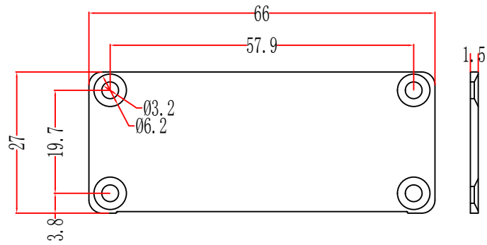
挡板
