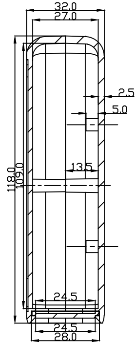
SECTION A-A
